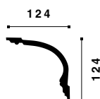
Z22 ARSTYL®
