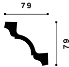
Z2 ARSTYL®
