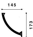
AD23 ARSTYL®
