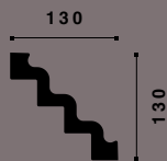
ST4 NOMASTYL®
