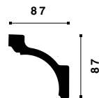
IL6 ARSTYL®
